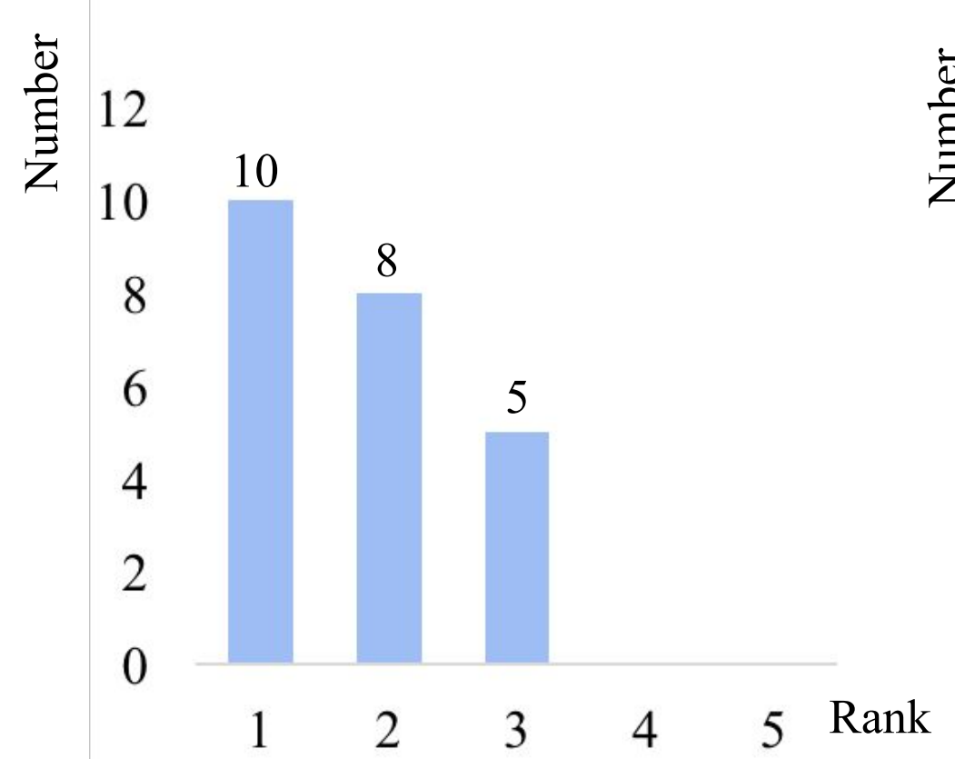
EnlightenGAN
