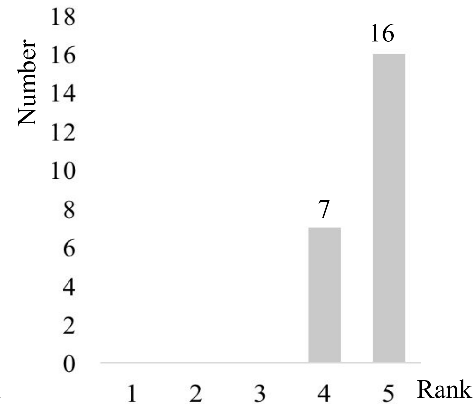
LIME
