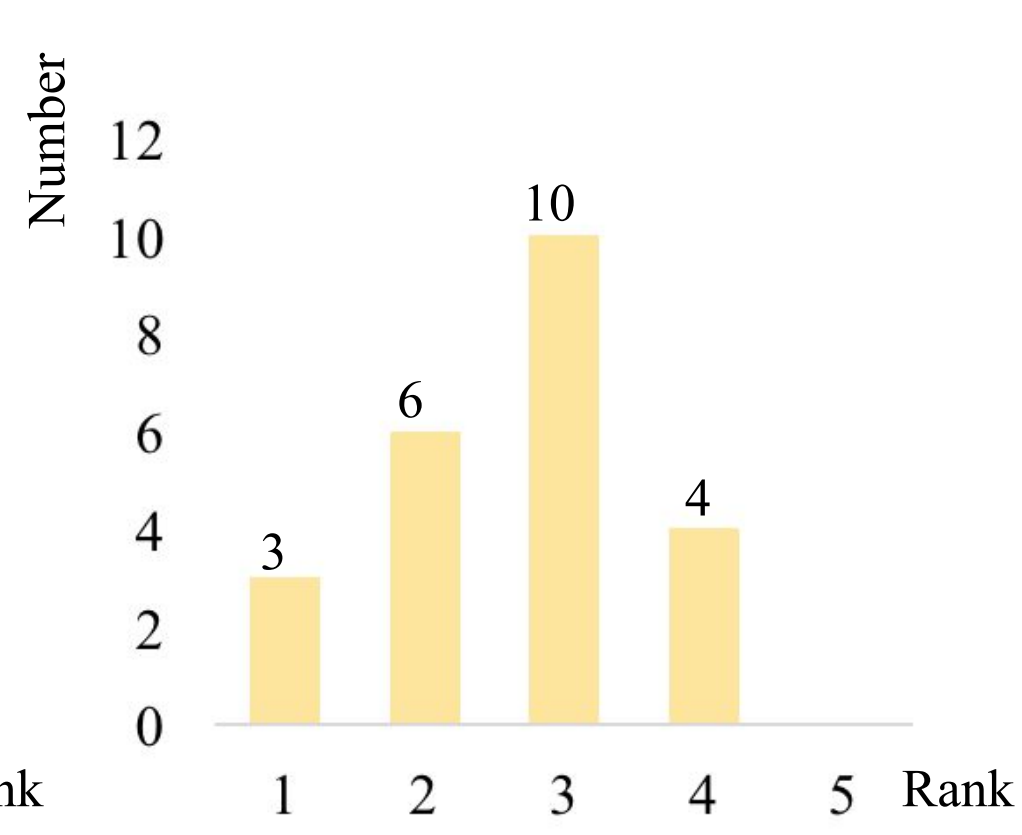
NPE
