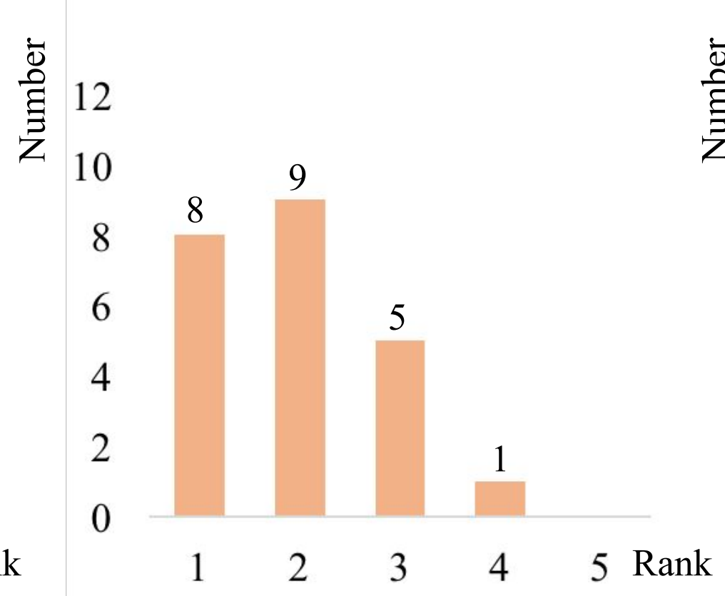
SRIE
